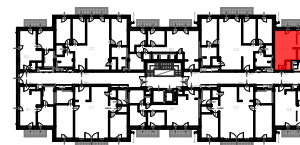
J2 ÉPÜLET 1. EMELET SZINTRAJZ
